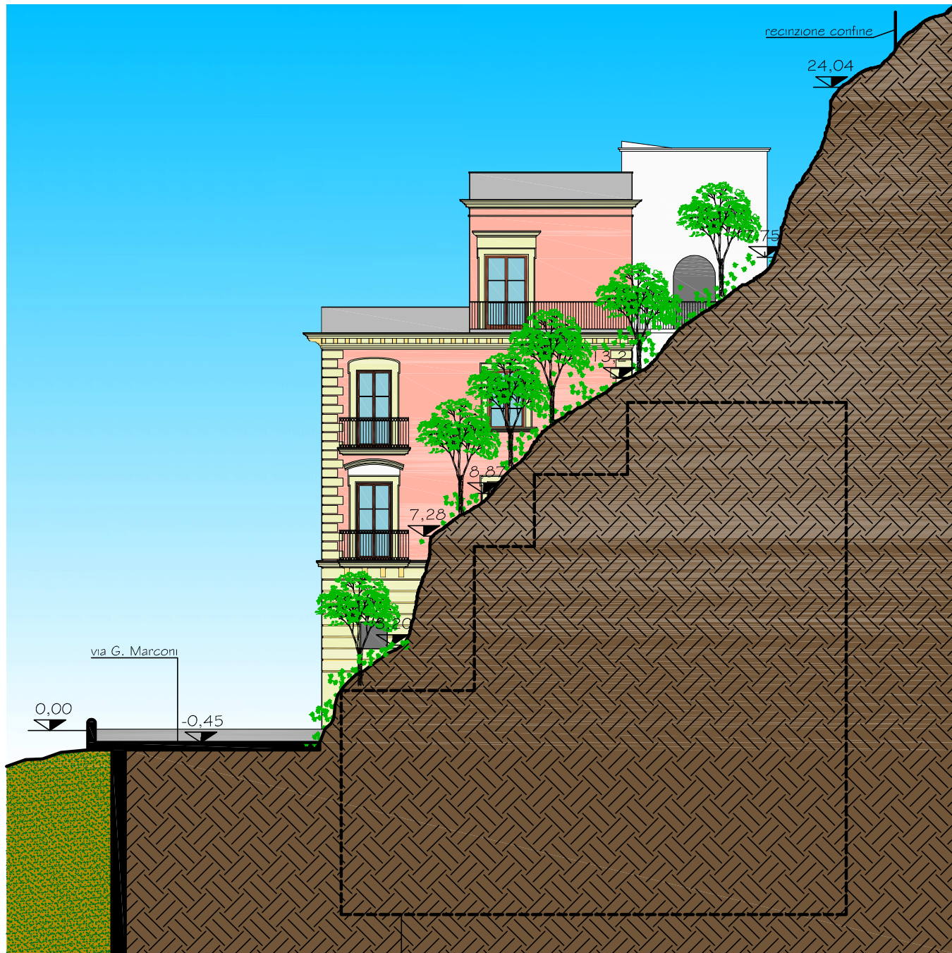
SEZIONE A-A Stato attuale
