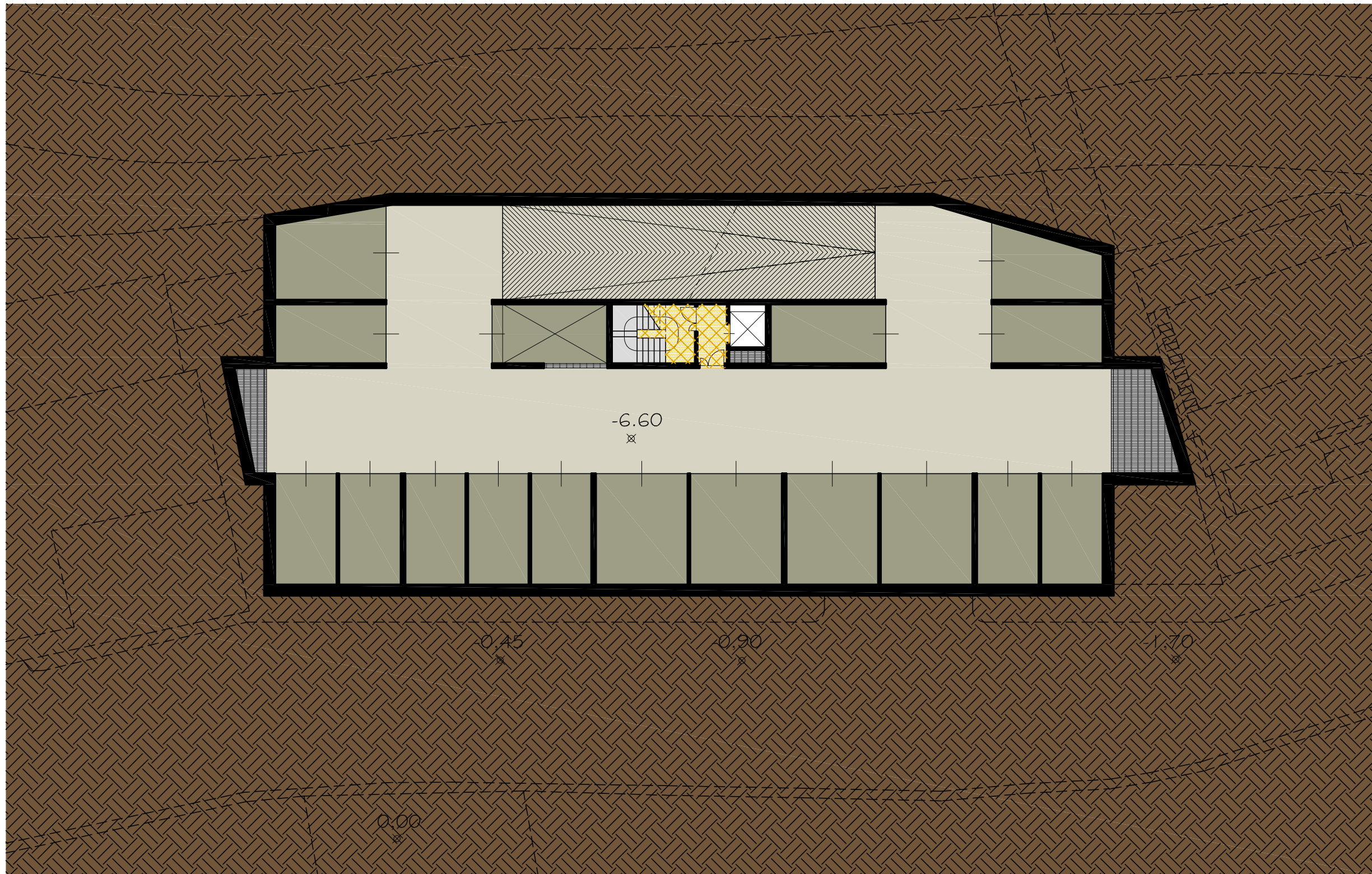
PIANTA A Q=-6.60
