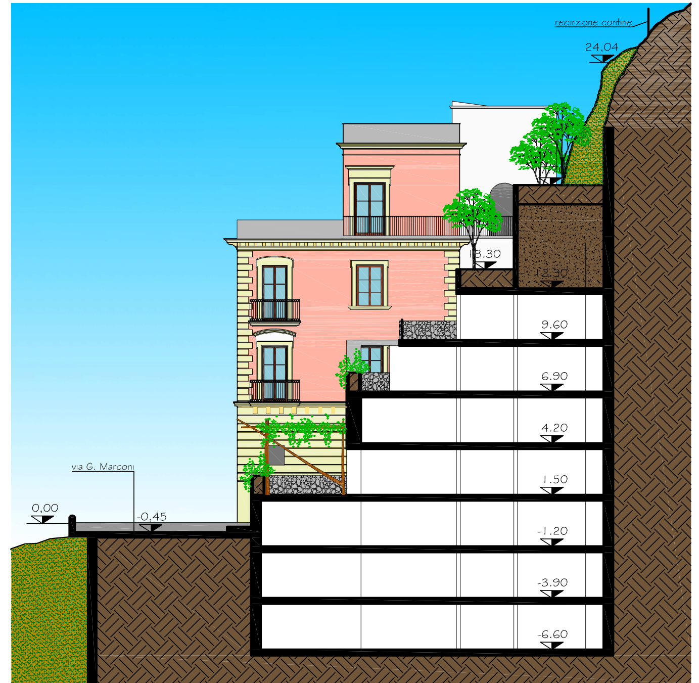
SEZIONE A-A Progetto
