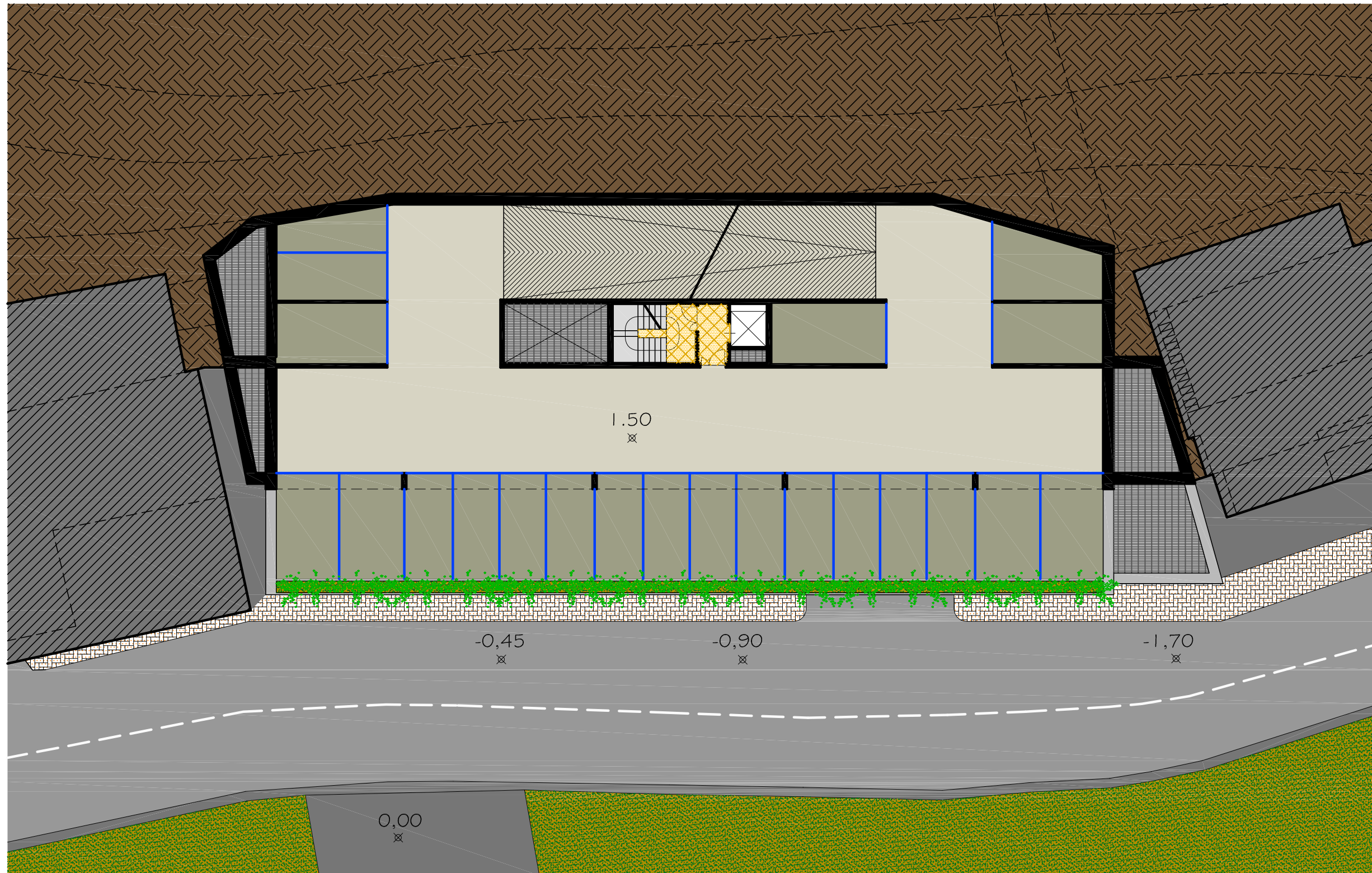
PIANTA A Q= 1.50
