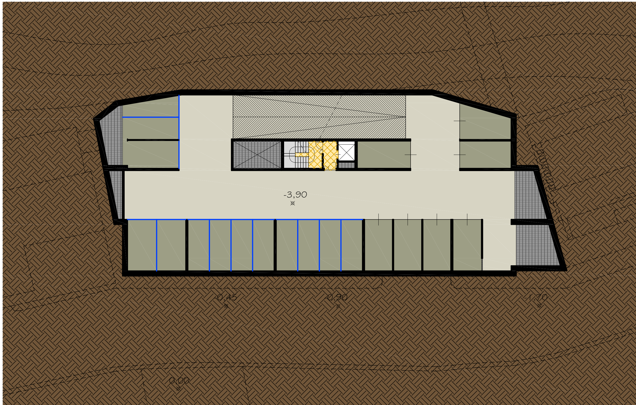
PIANTA A Q=-3,90
