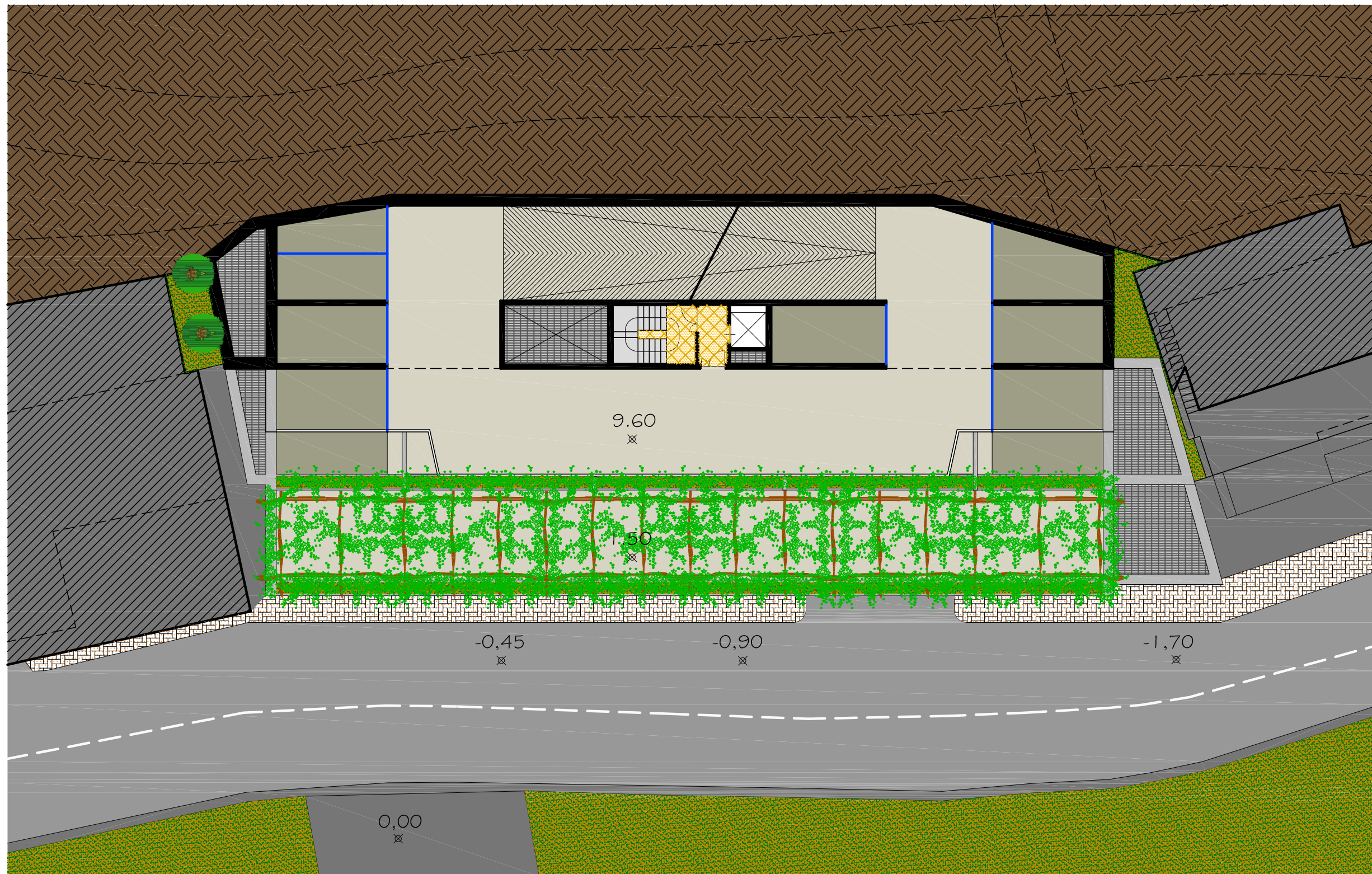
PIANTA A Q=9.60
